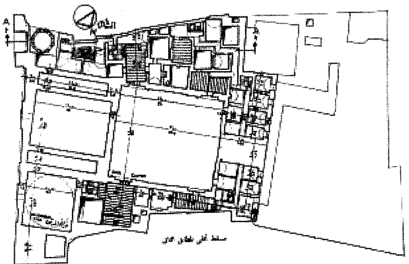
شكل رقم (٧): مدرسة الظاهر برقوق - مسقط أفقى للطابقين الأول والثانى.
